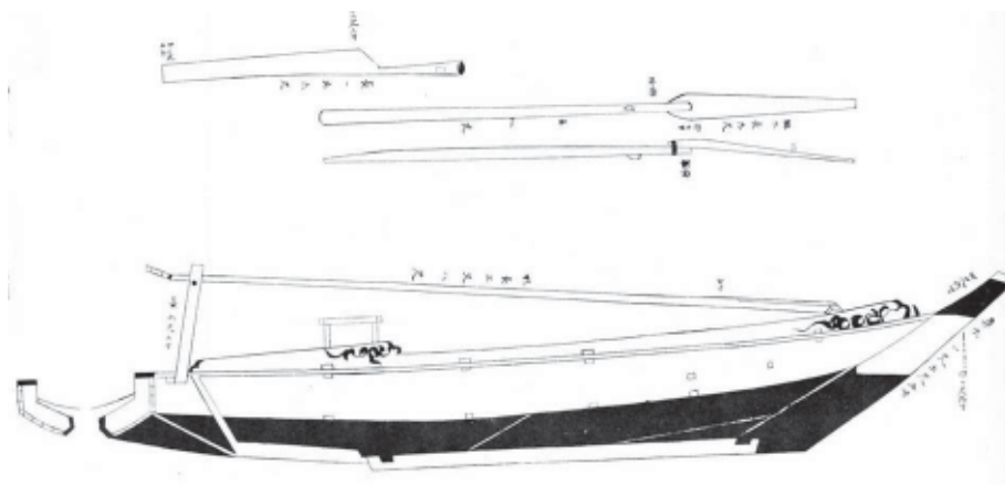
牛深の鰹釣船 総長 4丈2尺9寸 (約13mcm)
